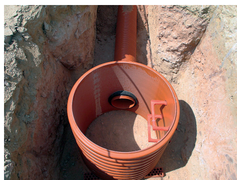
Acabado del fondo del pozo rematado con hormigón (Solamente recomendable sin freático)
