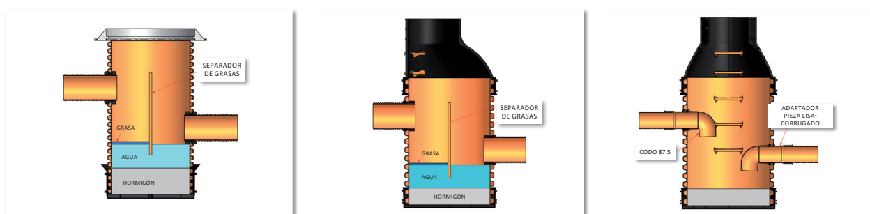
Arquetas y pozos separadores de grasas
