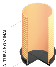
Pozo DN600 mm
