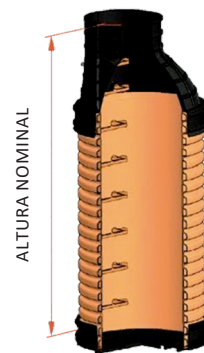
Pozos DN1000 y DN1200 mm
