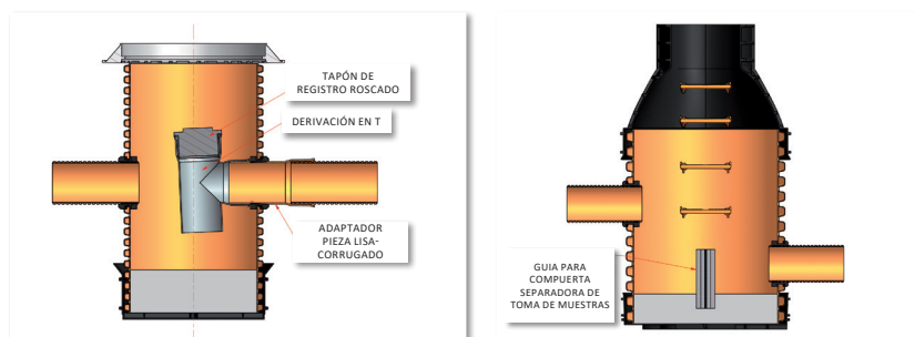
Arqueta sifónica
